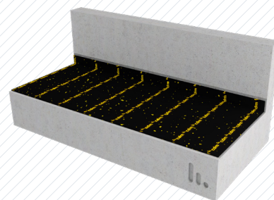
Sols non collés dalle en béton + pare-vapeur + Stravifloor Mat-F e
