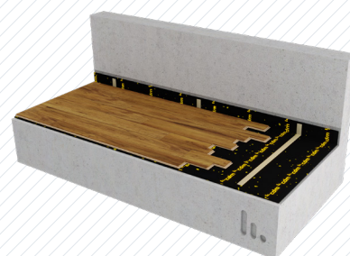
Sols non collés dalle en béton + pare-vapeur + Stravifloor Mat-F e (incl. joints scellés) + revêtement de finition
