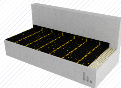
Sols collés dalle en béton + bande périmétrale + Stravifloor Mat-F e
