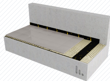
Sols collés dalle en béton + adhésif + Stravifloor Mat-F e + adhésif + revêtement de finition
