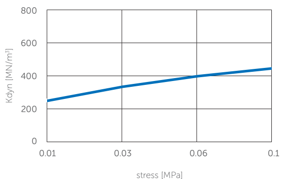
Rigidité dynamique
