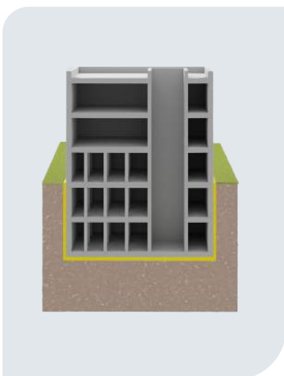
Figure 4.1 - Isolation de l'ensemble du bâtiment
